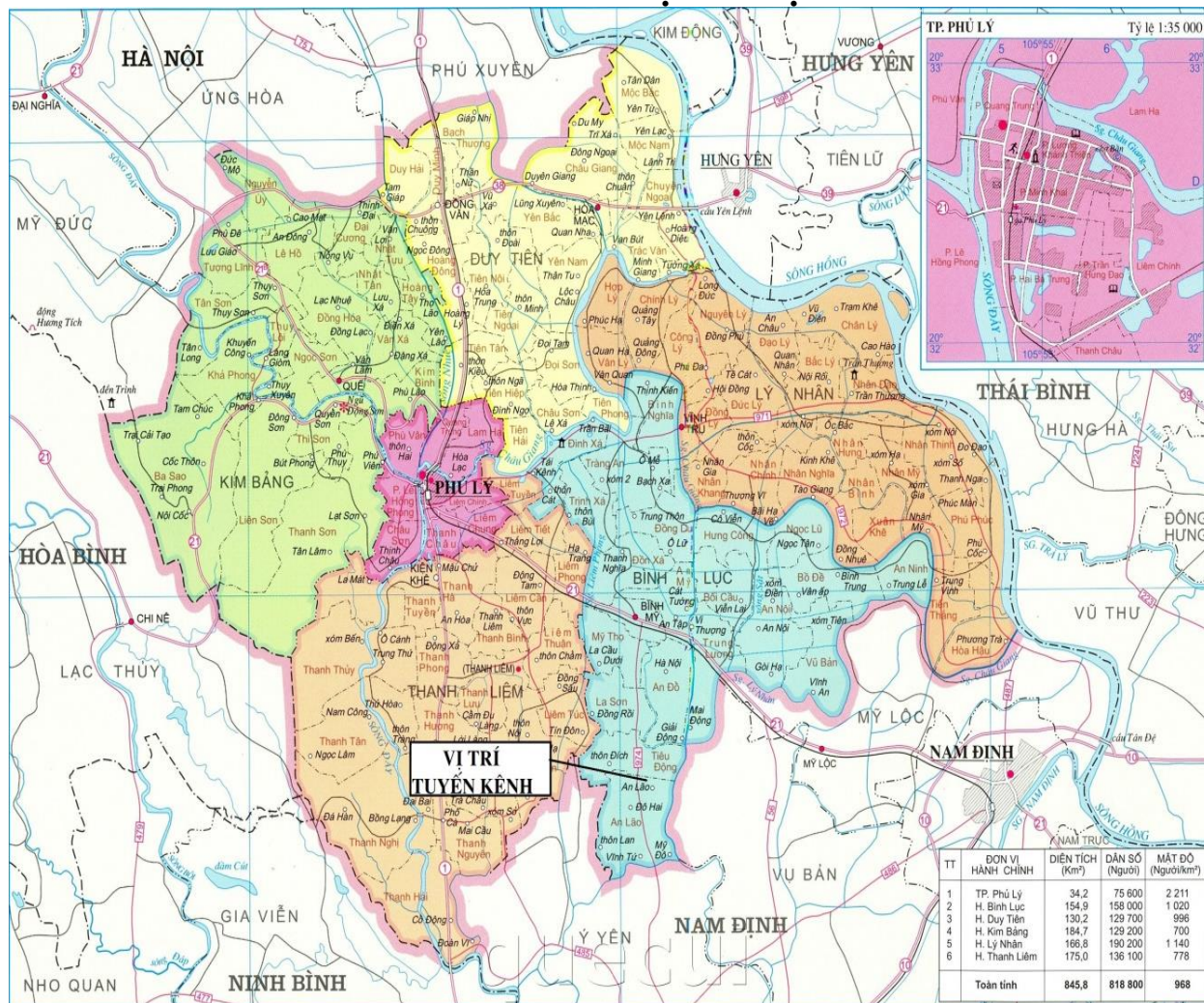
HÌNH 1.1 SƠ ĐỒ VỊ TRÍ DỰ ÁN
